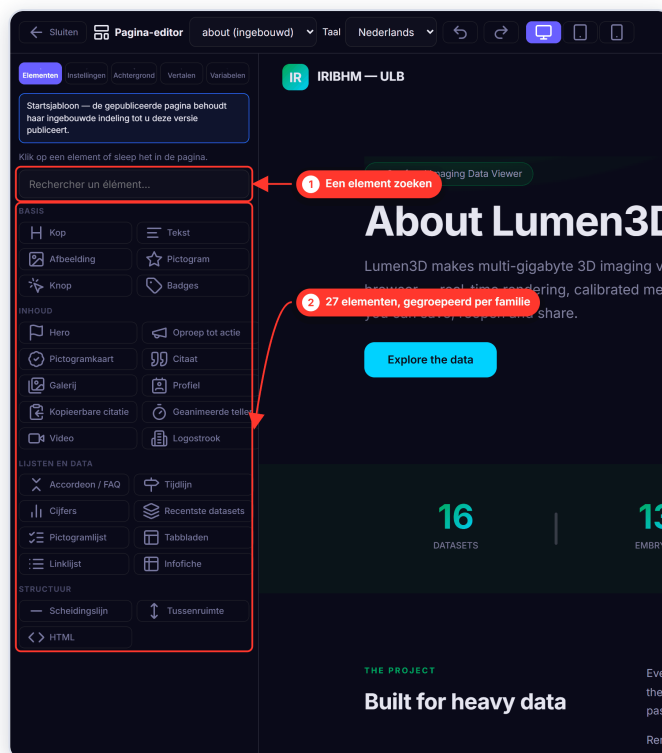
▲ Het elementenpalet.
