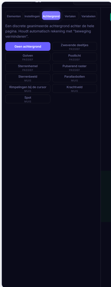
▲ Tabblad Achtergrond.
