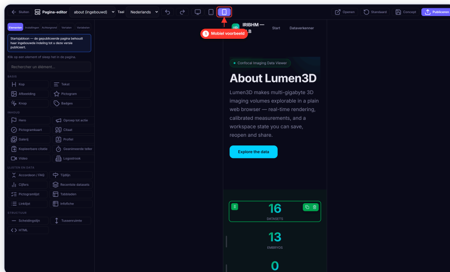
▲ Mobiel voorbeeld.
