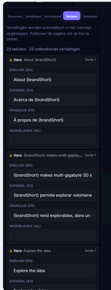
▲ Tabblad Vertalen.
