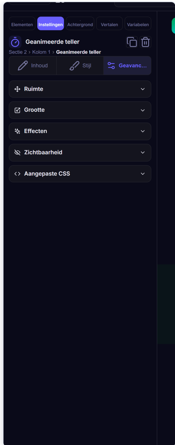
▲ Tabblad Geavanceerd.
