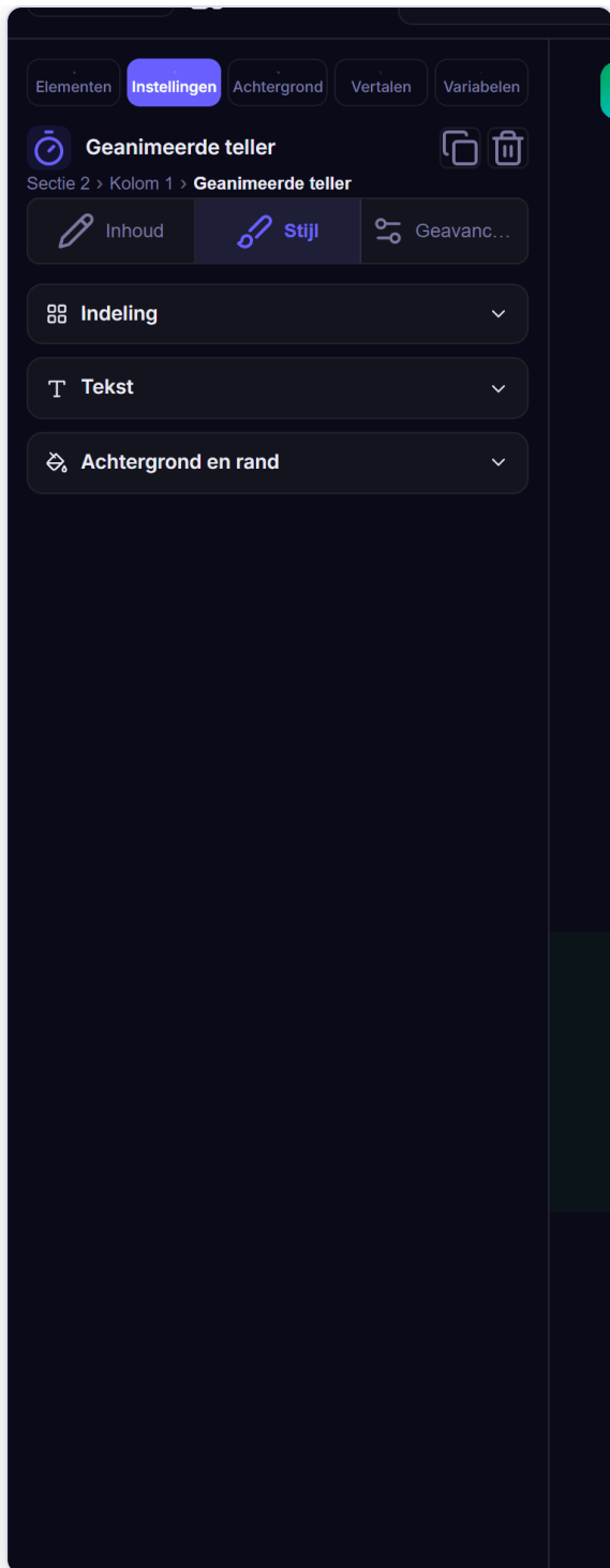
▲ Tabblad Stijl.
