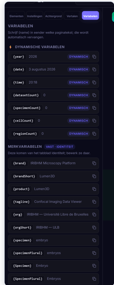
▲ Tabblad Variabelen.
